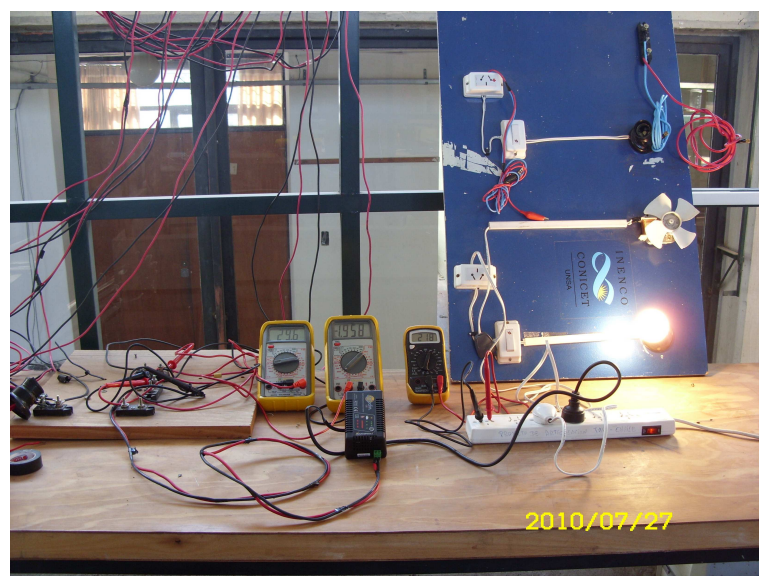
Figura 5: Dispositivo diseñado para la medida de la eficiencia del inversor.
