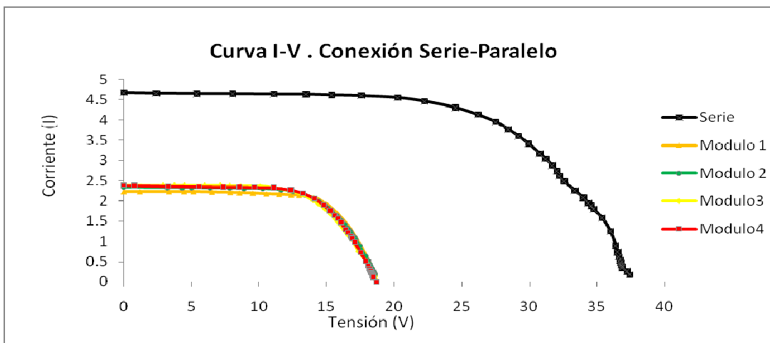
Figura 1: Caracterización de módulos fotovoltaicos. Conexión Serie-Paralelo
