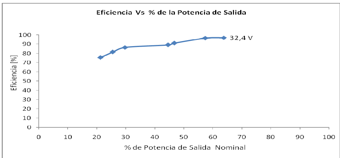
Figura 2: Eficiencia del inversor conectado a grupo electrógeno con tensión de entrada constante de 32.4V
