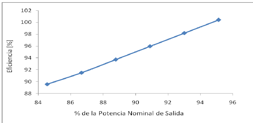
Figura 4: Eficiencia del Inversor conectado a la Red Eléctrica.
