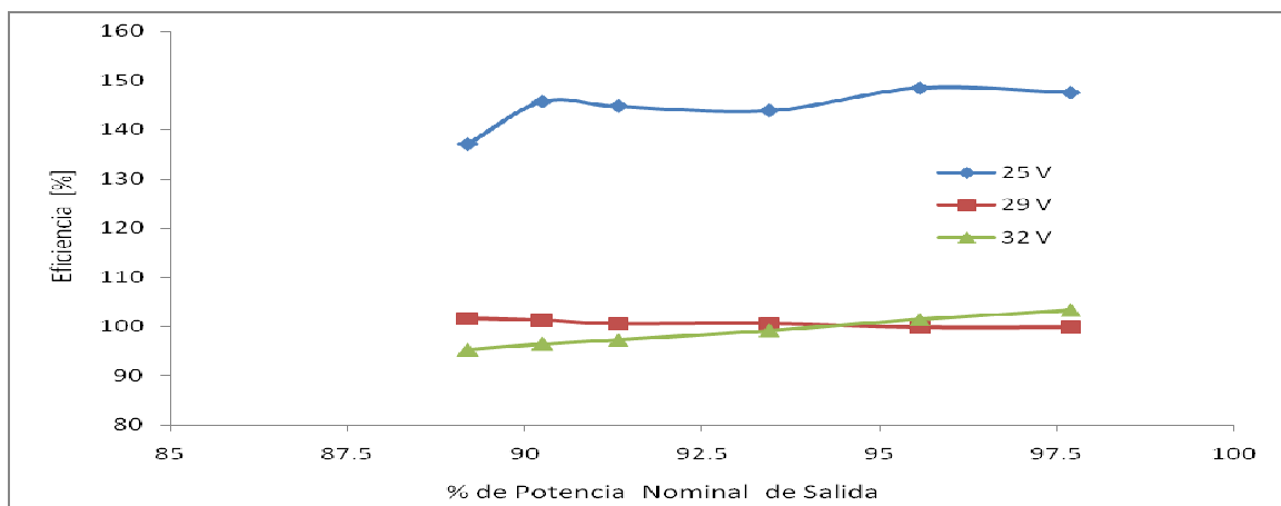
Figura 3: Eficiencia del Inversor conectado a Fuente Tensión. Para distintas tensiones de entrada
