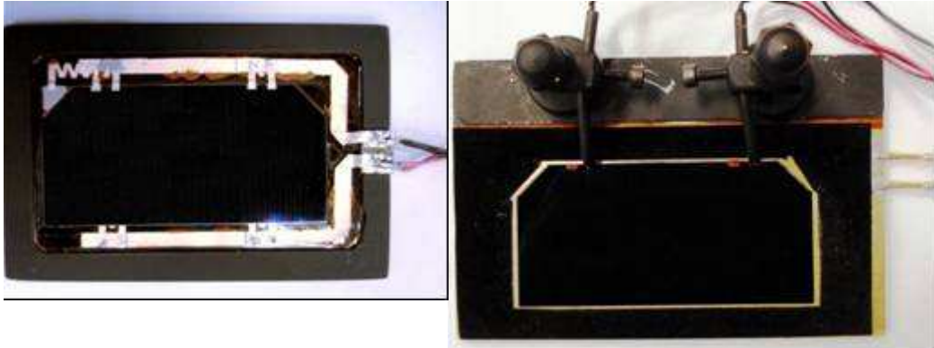
Figura 2: Izquierda, patrón secundario, celda ATJ CIC montada en un soporte de bronce pintado. Derecha, celda Emcore calibrada en la base del equipo de RE.
