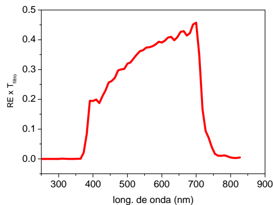
Figura 1. Transmitancia en función de la longitud de onda del filtro empleado en un radiómetro PAR de CNEA.
