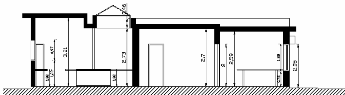
CORTE A-A
