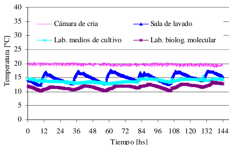
Figura 11. Temperaturas interiores del edificio.
