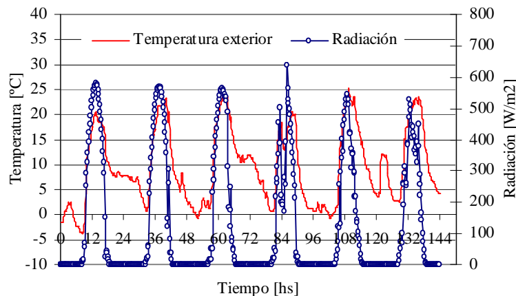
Figura 10. Radiación y temperatura exterior del tercer periodo.
