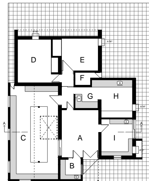
PLANTA GENERAL
