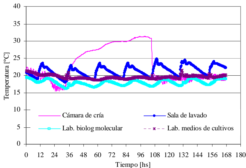
Figura 5. Temperatura en el interior del edificio Primer periodo.
