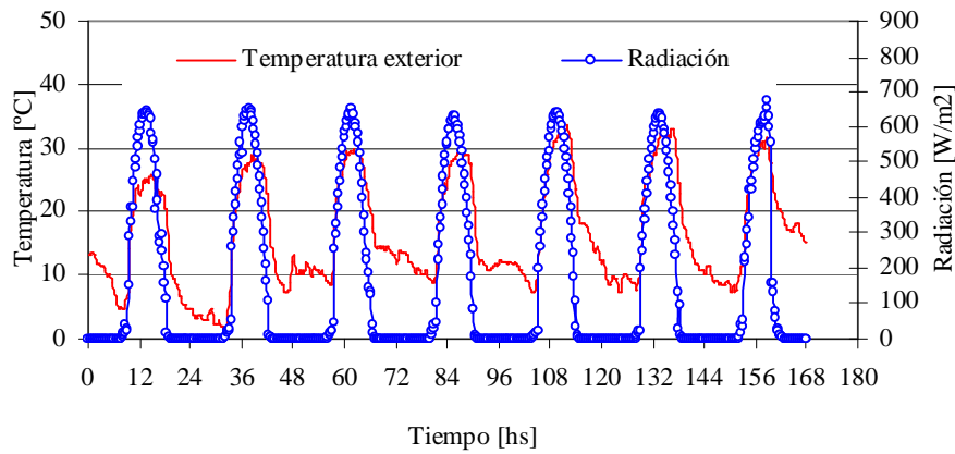
Figura 4. Temperatura y radiación exterior
