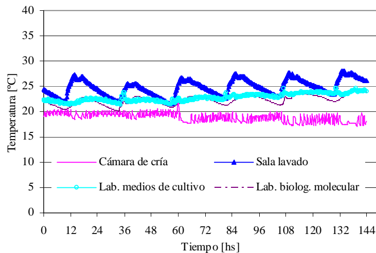
Figura 8. Temperaturas registras en el interior del edificio.
