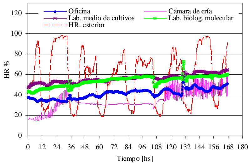
Figura 6. Humedad relativa exterior e interior de cuatro locales del edificio.
