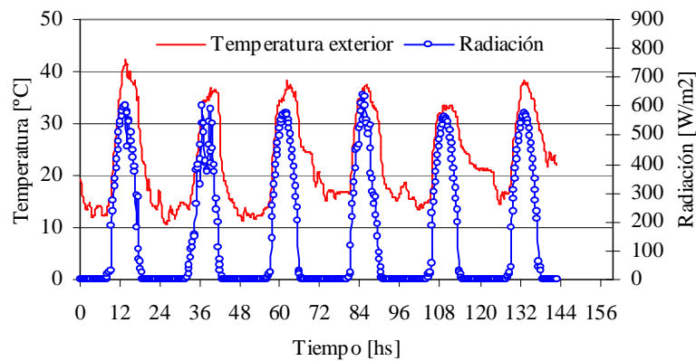
Figura 7. Radiación y temperatura exterior
