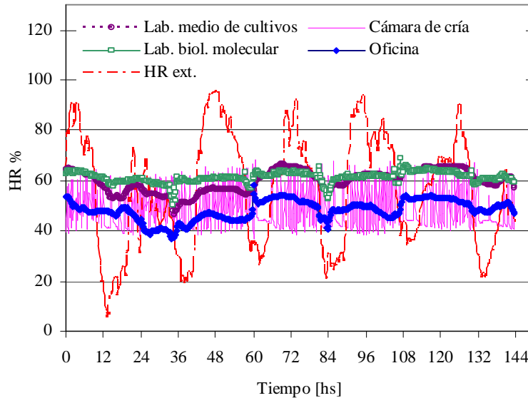
Figura 9. Humedad relativa interior y exterior para el segundo periodo
