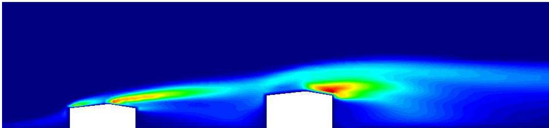
Figura 3: Energía Cinética Turbulenta ( v = 1.5 \text{ m/s} - \text{modelo } k - \epsilon )
