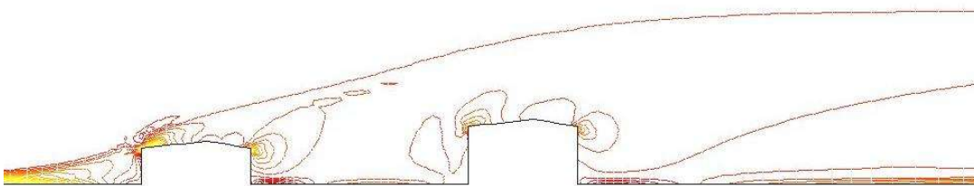
Figura 8: Líneas de Vorticidad ( v = 1.5 \text{ m/s} - modelo k - \omega )
