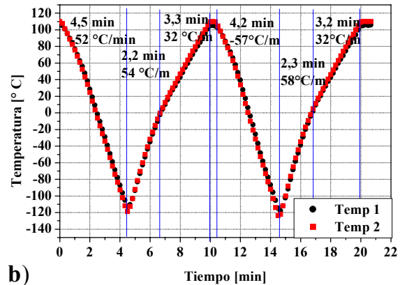
Figura 2: a) Temperatura del portamuestra con períodos de estabilización.. b) Ciclado térmico.
