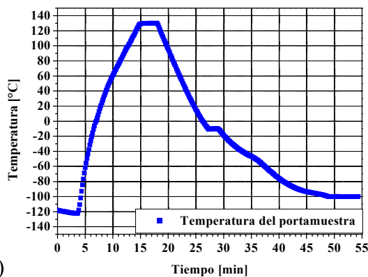
Figura 2: a) Temperatura del portamuestra con períodos de estabilización.. b) Ciclado térmico.
