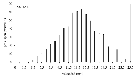
figura 3: distribución de la potencia meteorológica media disponible en función de la velocidad media horaria, para el año considerado.
