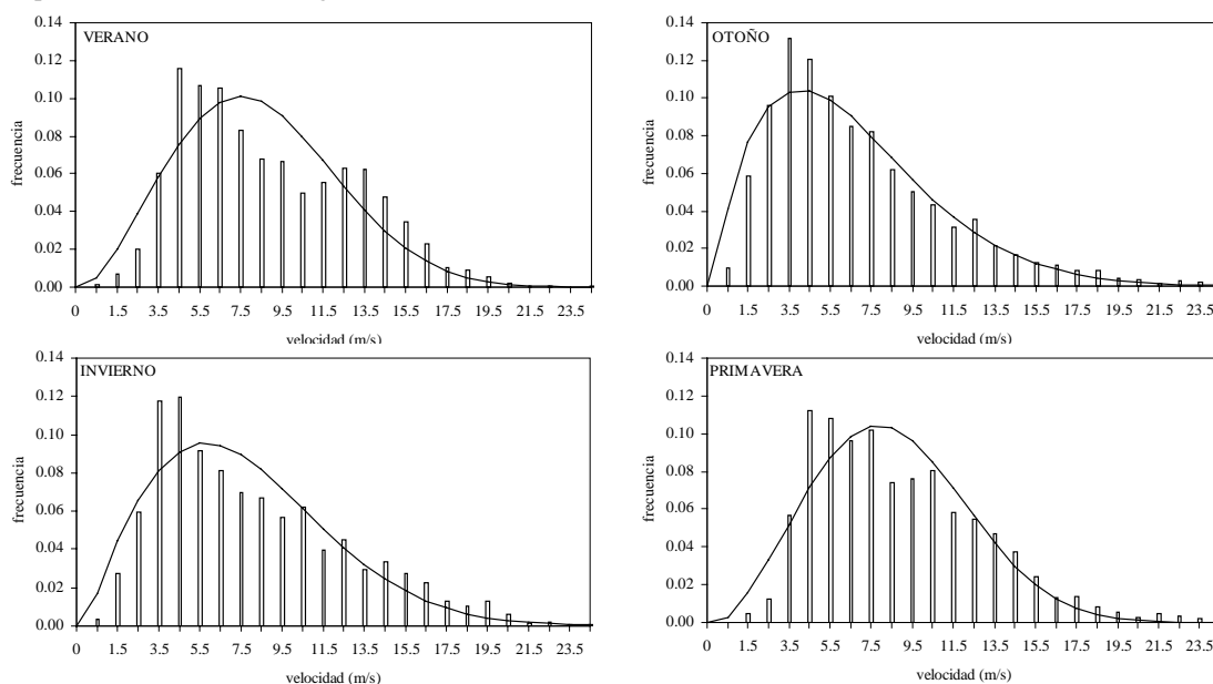
figura 1: distribución de frecuencias estacional de la velocidad media horaria del viento: las barras muestran los datos observados y la línea continua la distribución teórica de Weibull II.
