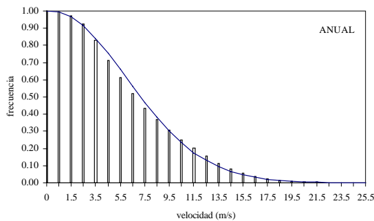
figura 2: distribución de frecuencias acumuladas de la velocidad media horaria del viento: las barras muestran los datos observados y la línea continua la distribución teórica.
