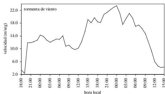
figura 5: comportamiento de la velocidad media durante una tormenta de viento, el eje de abscisas comienza el día 19/dic a las 18 horas y termina el 21/dic/95 a las 15 horas.
