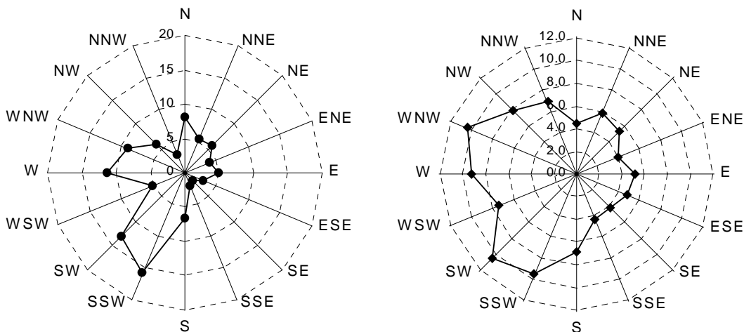
figura 4: a la izquierda rosa de los vientos indicando la frecuencia porcentual de las direcciones. A la derecha rosa de los vientos de intensidades expresadas en m/seg.
